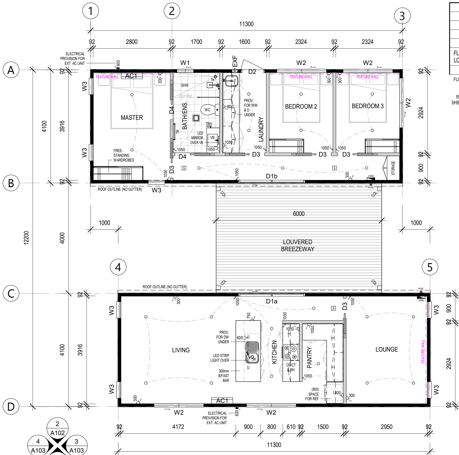
FLOOR PLAN 1 : 65
