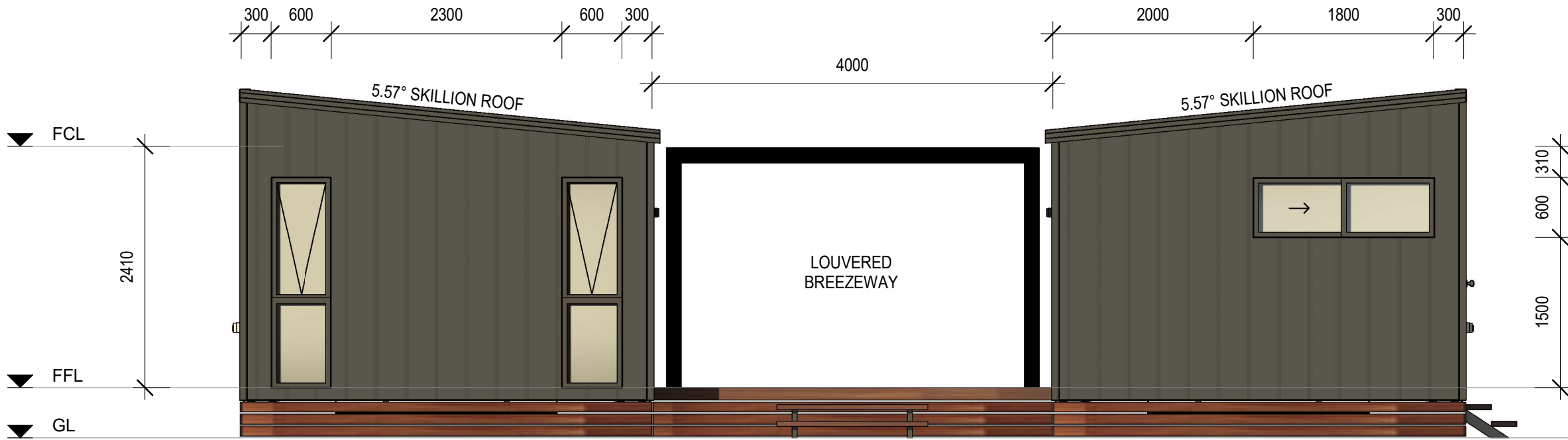
RIGHT ELEVATION (3)
