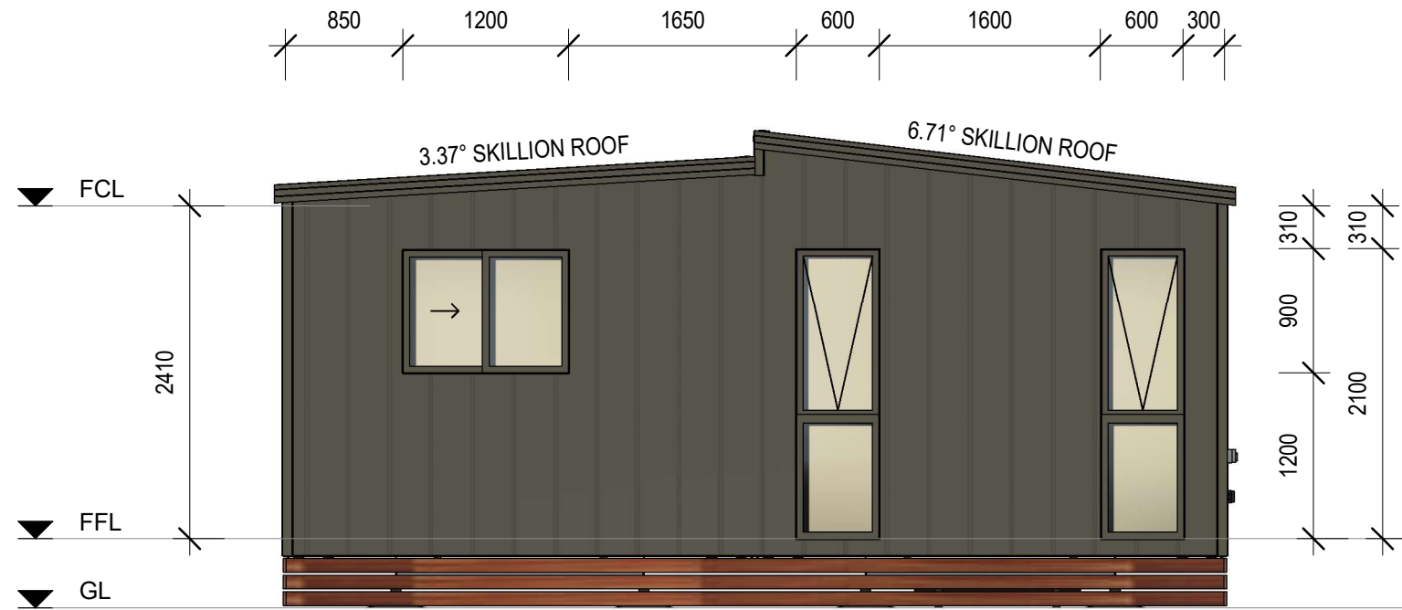
RIGHT ELEVATION (3)
