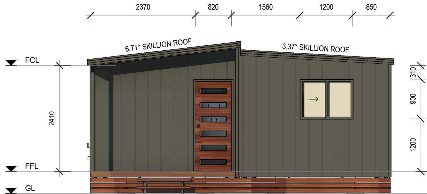
LEFT ELEVATION (4)
