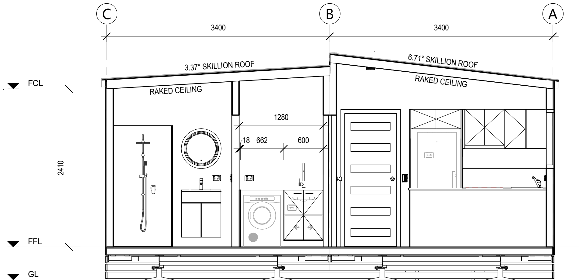
SECTION A-A
