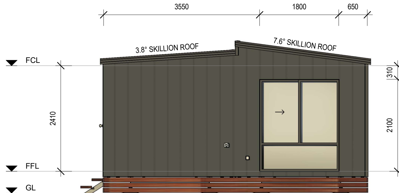
RIGHT ELEVATION (3)
