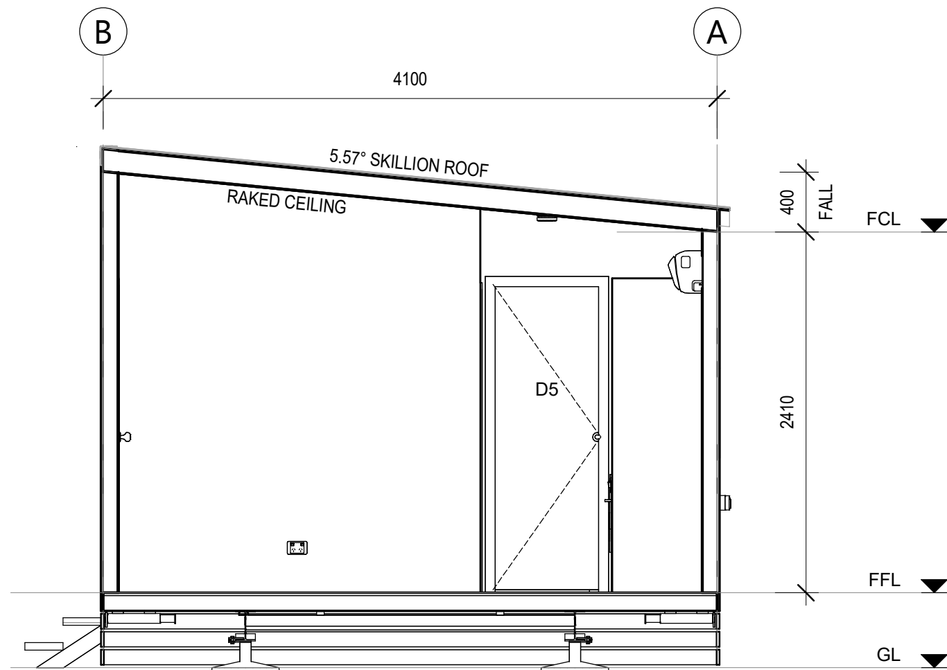
SECTION A-A
