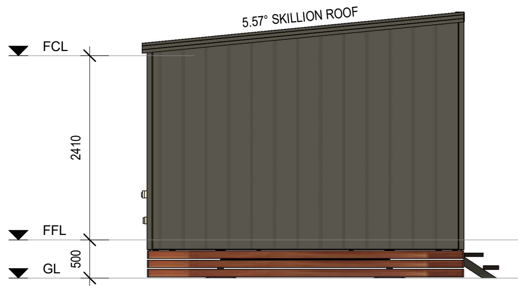
LEFT ELEVATION (4)
