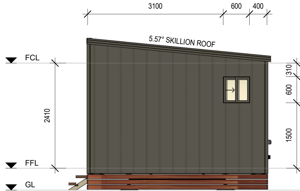
RIGHT ELEVATION (3)
