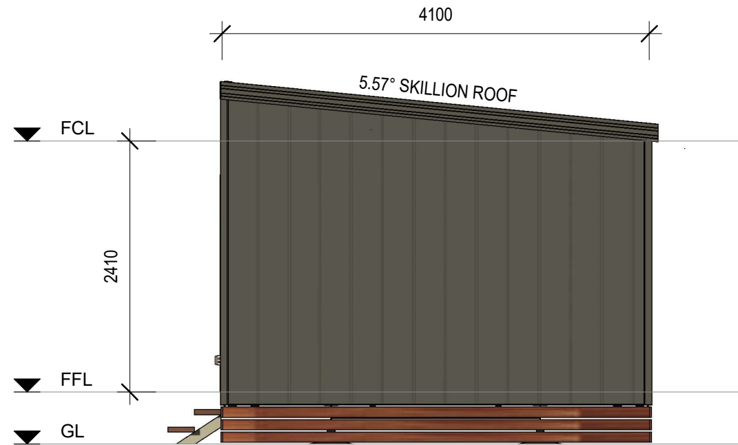
RIGHT ELEVATION (3)
